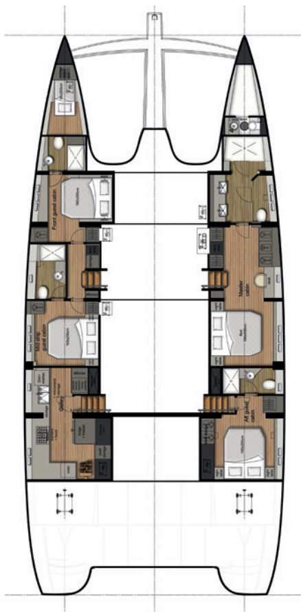
HULLS COQUES
